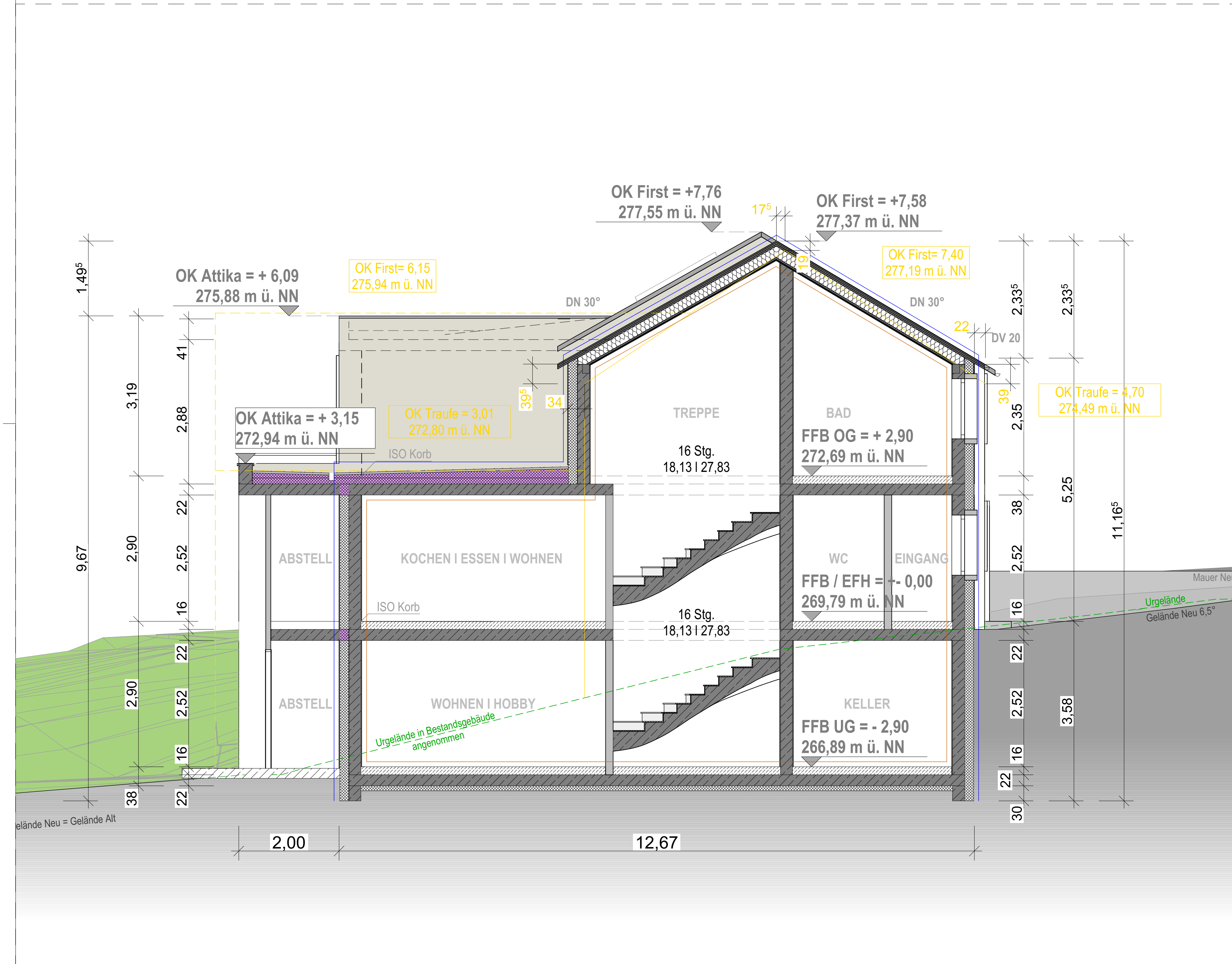
SCHNITT B_B M1:50
